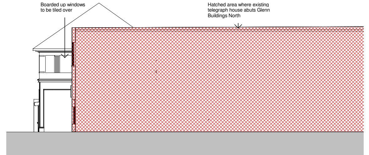
3 PBX_Existing Elevation DD 1 : 200
